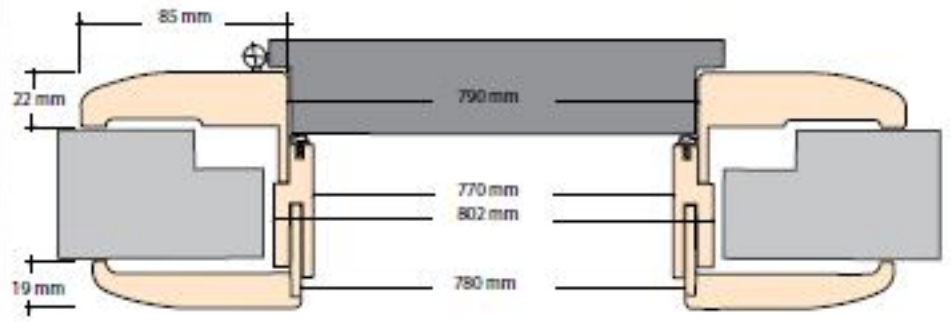
ITB-2 Renovierungszarge
