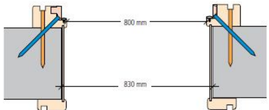
Blendrahmen mit Gegenbekleidung
