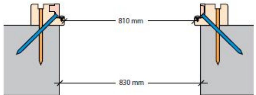
Blendrahmen
